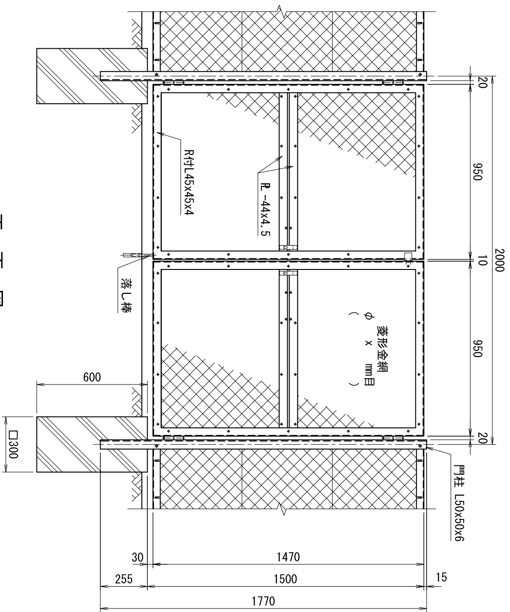
平面図 (S=1/20)
