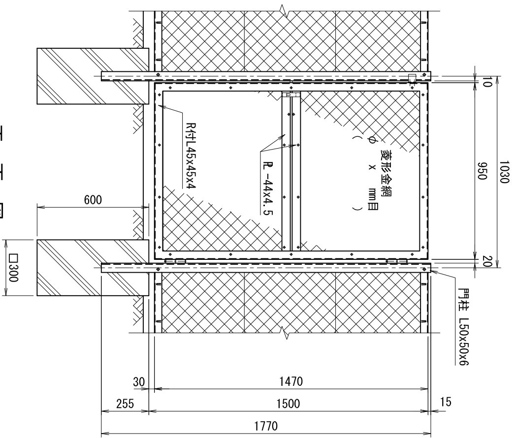
平面図 (S=1/20)
